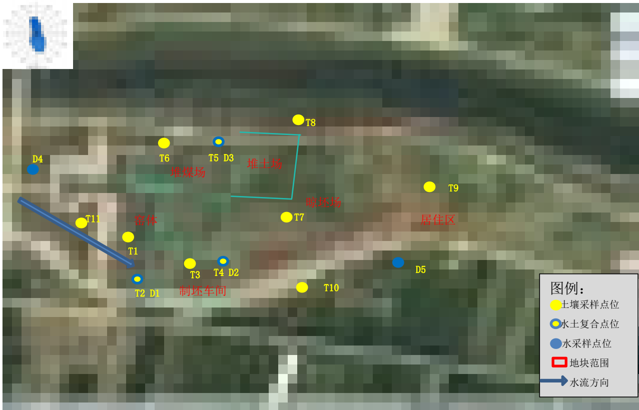
图 4.3-2 土壤和地下水监测布点图
