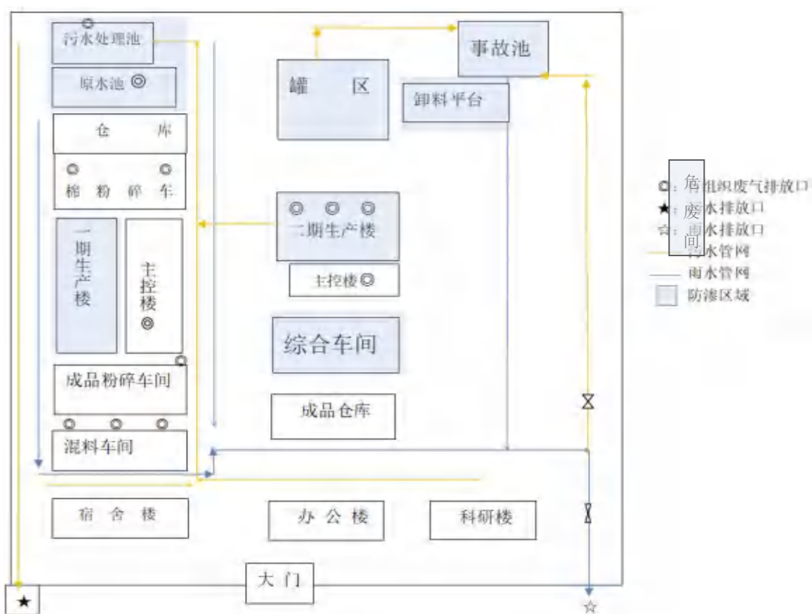
图 2.2-1 平面布置图
